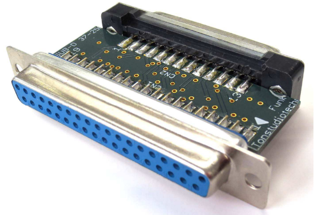
Ansicht Übergang zum SAM-3B.V2-Eingang
