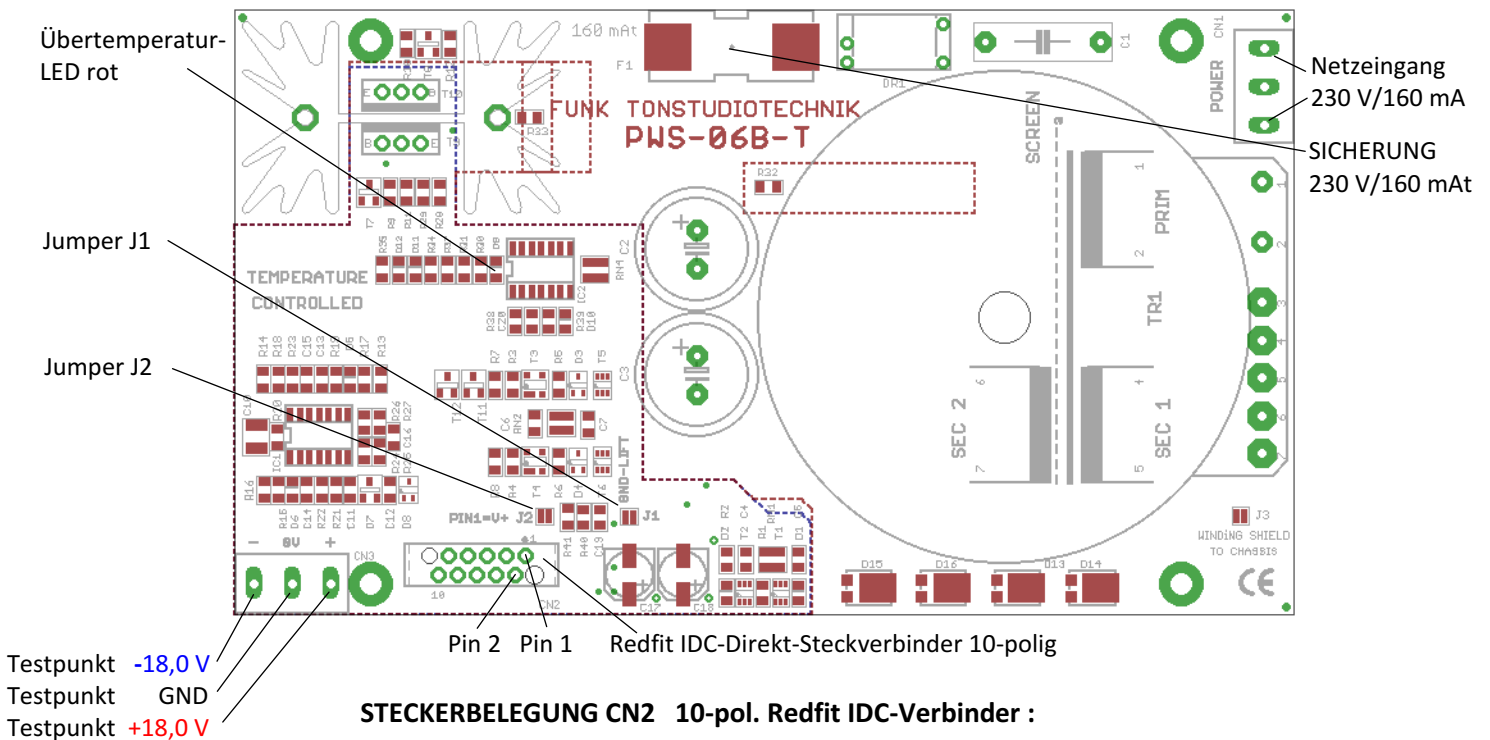
Leiterplatte PWS-06B-T Bauteile-Ansicht von oben in Originalgröße
