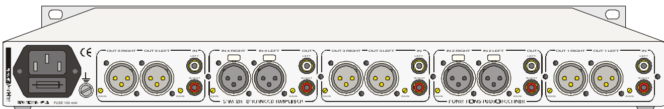
Rückansicht SAM-2A (Konfiguration 6 - 4 )
